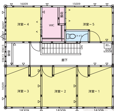
After 平面図2階
